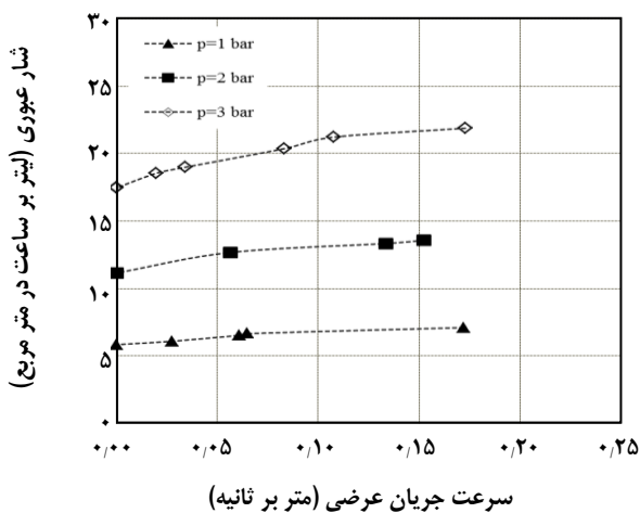
شکل ۳- تغییر شار عبوری به عنوان تابعی از سرعت جریان عرضی در فشارهای متفاوت برای غشای M2 در غلظت (الف) ۳۰۰۰، (ب) ۶۰۰۰ و (ج) ۹۰۰۰ میلی گرم بر لیتر.
