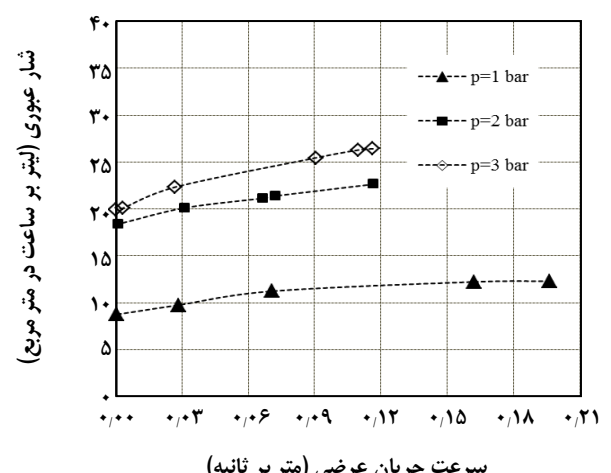
شکل ۲- تغییر شار عبوری به عنوان تابعی از سرعت جریان عرضی در فشارهای متفاوت برای غشای M1 در غلظت (الف) ۳۰۰۰، (ب) ۶۰۰۰ و (ج) ۹۰۰۰ میلی گرم بر لیتر.
