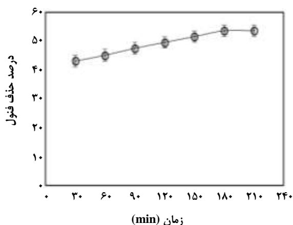
شکل ۱۰- نمودار تأثیر زمان بر درصد حذف فنول.
