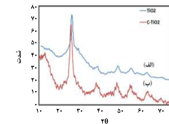
شکل ۲- الگوی پراش پرتو ایکس (الف) نانوذره‌های تیتانیای خالص (ب) نانوذره‌های تیتانیای آلیش یافته با کربن.
