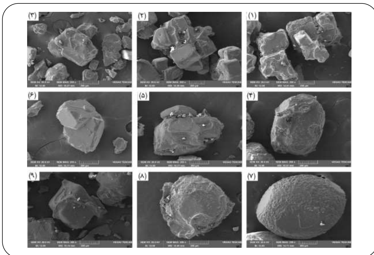
شکل ۲- تصویرهای میکروسکوپی بلورهای به دست آمده از آزمایش‌های نه‌گانه تاگچی با بزرگنمایی ۲۵۰ برابر. اعداد شکل‌ها متناظر با شماره آزمایش‌ها است.
