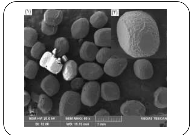
شکل ۸ - تصویرهای میکروسکوپی بلورهای آمونیوم پرکلرات نمونه بهینه. (۱) بزرگنمایی ۵۰ برابر، (۲) بزرگنمایی ۱۵۰ برابر.
