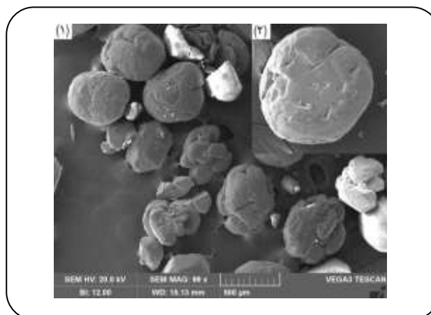
شکل ۱- تصویرهای میکروسکوپی بلورهای آمونیوم پرکلرات صنعتی. (۱) بزرگنمایی ۹۹ برابر، (۲) بزرگنمایی ۲۰۰ برابر.
