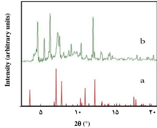
شکل ۸ - طیف XRD شبیه سازی شده با استفاده از داده‌های بلور نگاری (a) و نانو ذره‌های سنتز شده (b).
