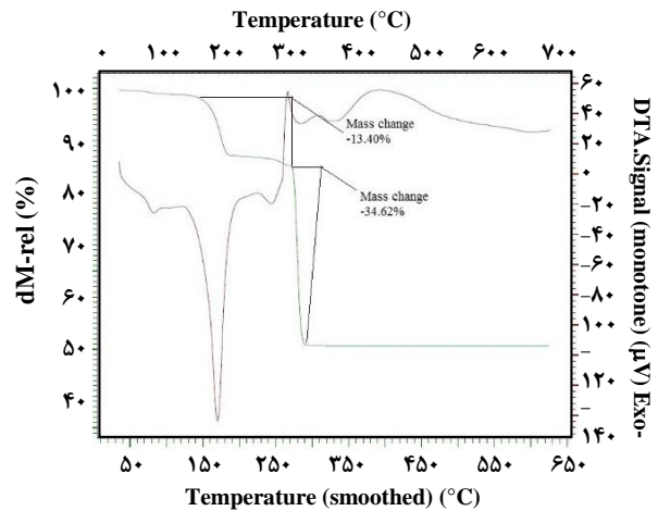
شکل ۹ - منحنی تجزیه گرمایی کمپلکس [\text{Cu}(\text{DPC})(\text{H}_2\text{O})_3] .
