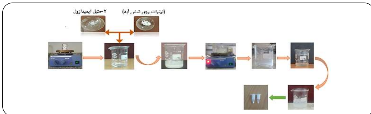
شکل ۳- مرحله‌های سنتز نانوذره‌های ZIF-8 با مایع‌های یونی.
