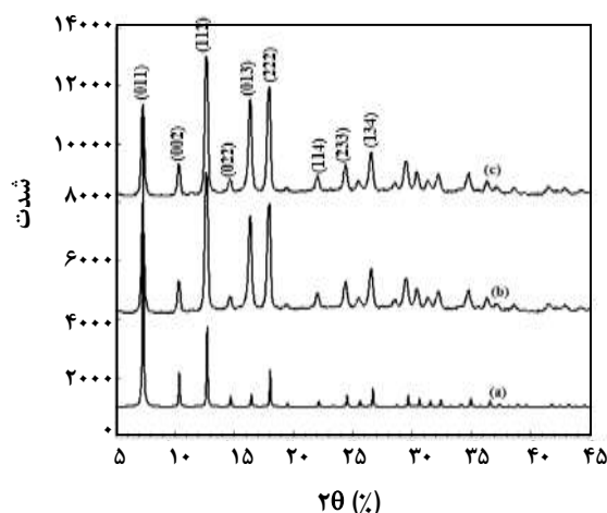
شکل ۶ - الگوی پراش پرتو ایکس، ZIF-8 شبیه سازی شده، (a) ZIF-8 سنتز شده با نسبت مولی فلز به اتصال دهنده ۱ به ۸ (b) نسبت مولی ۱ به ۴.
