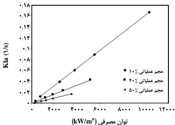
شکل ۵ - مقادارهای K_{La} محاسبه شده بر اساس معادله‌ی (۶) بر حسب توان مصرفی در راکتور زیستی نیمه‌صنعتی ۵۰ لیتری با قطر داخلی ۳۶ سانتی‌متر ( L/D=1/37 ).
