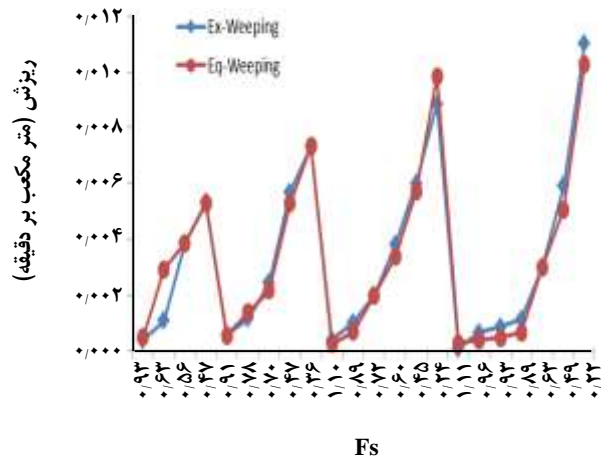
شکل ۱۳- نمودار مقایسه‌ای نتیجه‌های به دست آمده از ریزش در کار تجربی و معادله تجربی.
