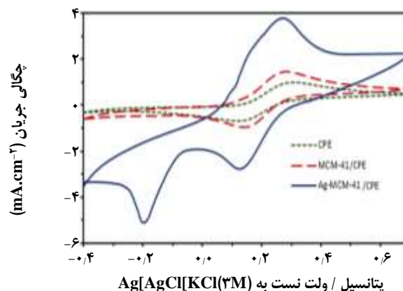
شکل ۴- ولتاموگرام چرخه‌ای الکترودهای CPE، MCM-41/CPE و Ag-MCM-41/CPE در محلول فری سیانید ۱۰ میلی مولار و ۰/۱ مولار KCl در سرعت اسکن ۲۰ mV/s.
