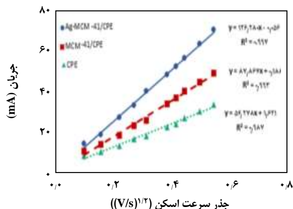
شکل ۵ - نمودار تغییرهای جریان پیک آندی الکترودها بر حسب جذر سرعت اسکن در محلول ۱ میلی مولار پتاسیم فری سیانید در \text{pH} = 7 و الکتروپولیت ۰/۱ مولار پتاسیم کلرید (سرعت اسکن ۵-۳۰ میلی ولت بر ثانیه).
