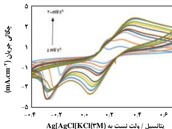
شکل ۹- ولتاموگرام چرخه ای الکتروکد Ag-MCM-41/CPE در سرعت اسکن ۵ تا ۳۰ میلی ولت بر ثانیه با غلظت ۰/۰۱ مولار فرمالدهید.
