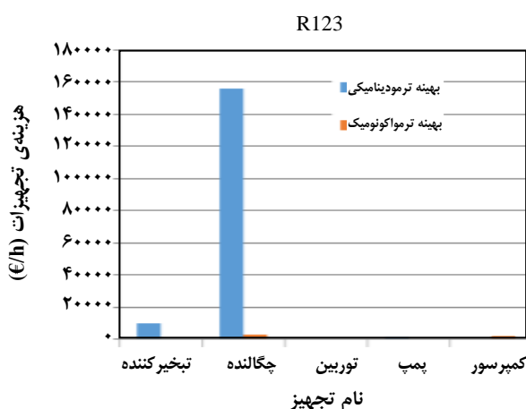
نمودار ۱۷- سهم هر یک از تجهیزها در هزینه کل سامانه در طراحی بهینه ترمودینامیکی و ترموآکونومیک - سیال R123 (بدون احیاکننده).
