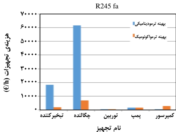
نمودار ۱۵- سهم هر یک از تجهیزها در هزینه کل سامانه در طراحی بهینه ترمودینامیکی و ترموآکونومیک- سیال R245fa (بدون احیاکننده).
