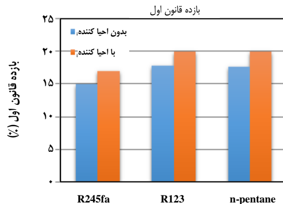
نمودار ۷- بازده قانون اول در طراحی بهینه ترمودینامیکی.
