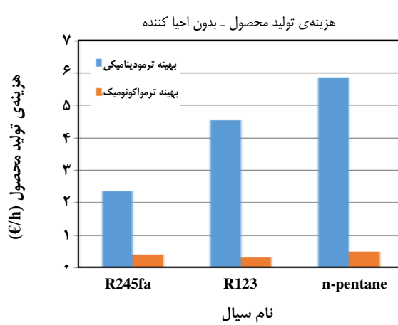
نمودار ۱۴- نمودار مربوط به هزینه ی تولید محصول چرخه برای بهینه سازی ترمودینامیکی و ترموآکونومیک - چرخه با احیاکننده.
