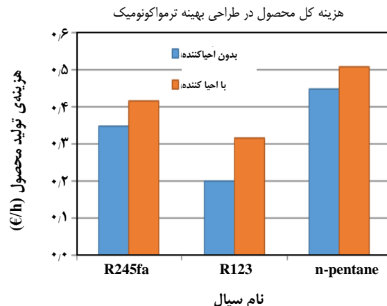
نمودار ۱۲- هزینه کل محصول در طراحی بهینه ترموآکونومیک در دو حالت بدون مبدل احیا کننده و با احیاکننده.
