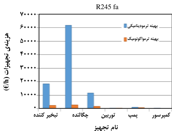
نمودار ۱۶ - سهم هر یک از تجهیزها در هزینه کل سامانه در طراحی بهینه ترمودینامیکی و ترموآکونومیک- سیال R245fa (با احیاکننده).
