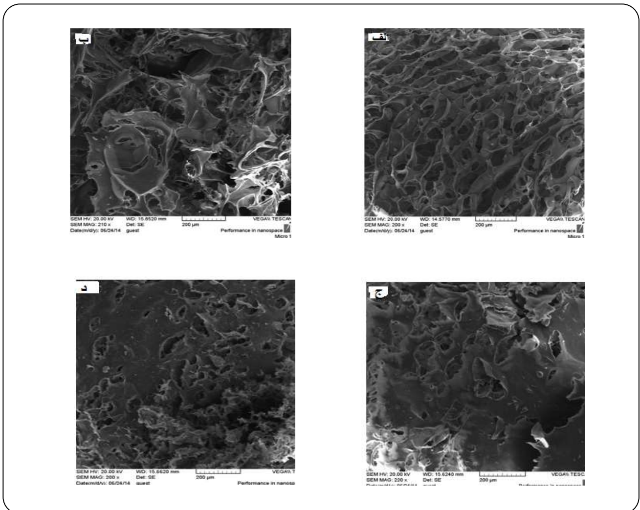
شکل ۴- ریزنگار میکروسکوپ الکترونی رویشی از دانه کیتوسان با بزرگنمایی ۲۰۰ برابر الف) بدون نانوذره های گرافن عامل دار شده (ب) دارای ۱٪ وزنی گرافن عامل دار شده، ج) دارای ۲٪ وزنی گرافن عامل دار شده و د) دارای ۵٪ وزنی گرافن عامل دار شده.
