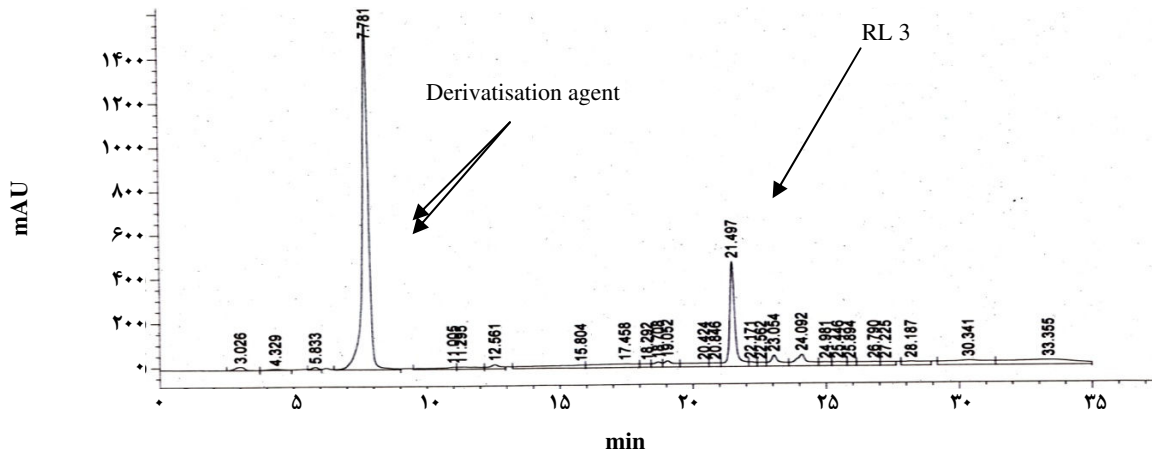
شکل ۱۰- نمونه‌ای از نتیجه‌های دستگاه HPLC در مورد تزریق رامولیبید ۳ به تنهایی.
