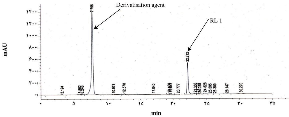
شکل ۱۱- نمونه‌ای از نتیجه‌های دستگاه HPLC در مورد تزریق رامولیبید ۱ به تنهایی.
