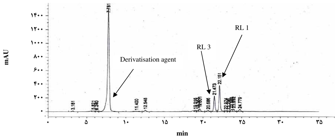
شکل ۱۲- نمونه‌ای از نتیجه‌های دستگاه HPLC در مورد تزریق رامولیبید تولید شده در این پژوهش.
