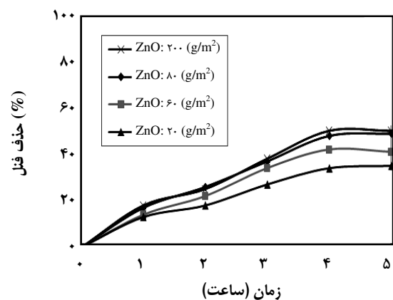
شکل ۱۱- تأثیر مقدار ماده کاتالیست روی بازده حذف سامانه. (غلظت فنل ۱۰۰ میلی‌گرم در لیتر، pH برابر ۷ و توان لامپ ۸ وات).
