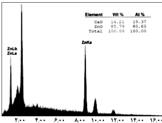
شکل ۴- نتیجه‌های تجزیه EDAX بتن پوشش یافته با ZnO. (سطح بتنی به روش WS آماده سازی شده است).
