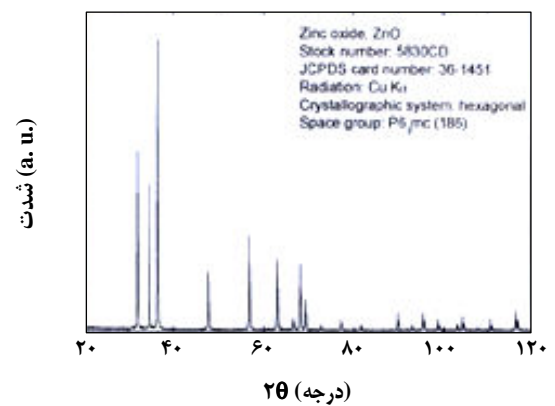
شکل ۵- نتایج آزمایش XRD نانو ذرات روی اکسید به قطر ۵۰ نانومتر. (سطح بتنی به روش WS آماده سازی شده است).
