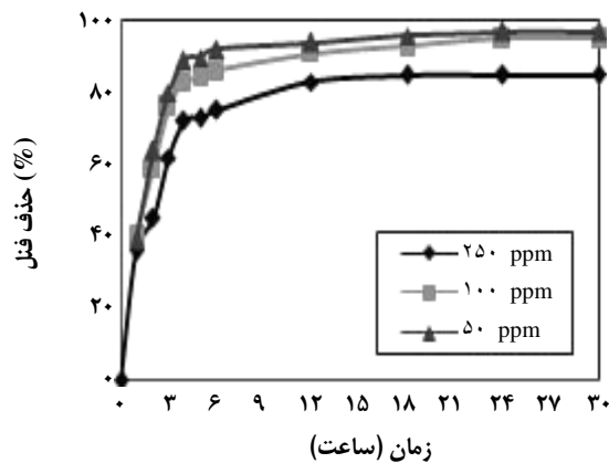
شکل ۱۲- بازده حذف سامانه در شرایط بهینه برای غلظت‌های گوناگون فنل.
