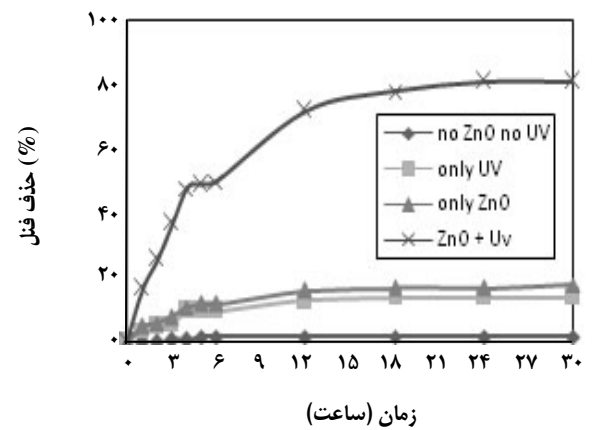
شکل ۶- راندمان حذف فنل در شرایط گوناگون مورد مطالعه. (غلظت فنل ۱۰۰ میلی گرم بر لیتر، pH برابر ۷، توان لامپ ۸ وات و کاتالیست ۸۰ گرم بر متر مربع) (سطح بتنی به روش WS آماده سازی شده است).
