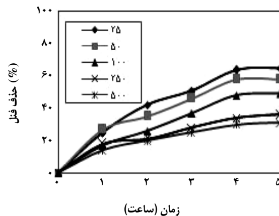
شکل ۸- تأثیر غلظت فنل روی بازده حذف سامانه. (pH برابر ۷، توان لامپ ۸ وات، و میزان کاتالیست ۸۰ گرم بر متر مربع).
