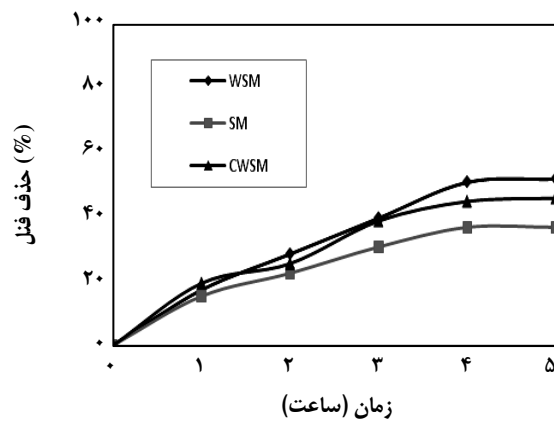
شکل ۷- تأثیر روش تثبیت روی بازده حذف سامانه. (غلظت فنل ۱۰۰ میلی گرم در لیتر، pH برابر ۷، توان لامپ ۸ وات و کاتالیست ۸۰ گرم بر متر مربع).
