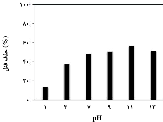
شکل ۹ - تأثیر pH روی بازده حذف سامانه. (غلظت فنل ۱۰۰ میلی گرم در لیتر، لامپ ۸ وات و کاتالیست ۸۰ گرم بر متر مربع).
