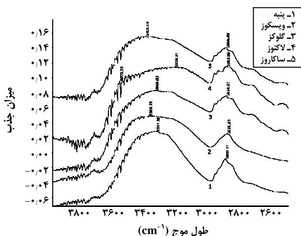
شکل ۲- ناحیه 4000-2500 \text{ cm}^{-1} نمونه‌های سلولزی شامل پنبه، ویسکوز و سلولز میکروبی تولید شده از سه محیط کشت حاوی گلوکز، لاکتوز و ساکاروز.
