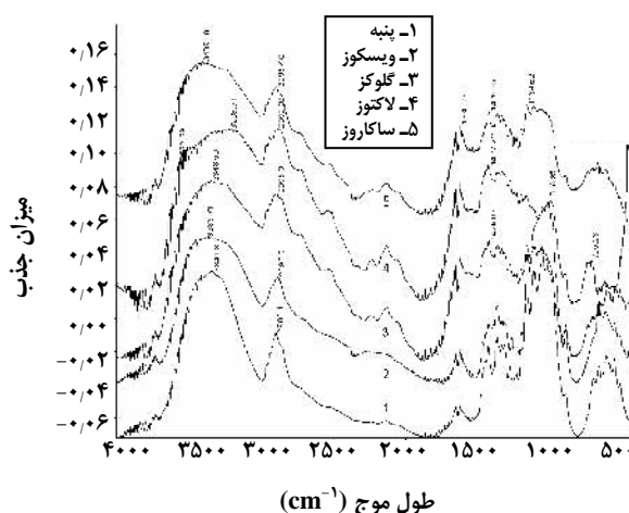
شکل ۳- طیف‌های فرو سرخ لیف‌های پنبه، ویسکوز و سلولز میکروبی تولید شده از سه محیط کشت حاوی گلوکز، لاکتوز و ساکاروز.
