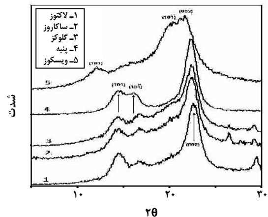
شکل ۸ - طیف های پراش اشعه ایکس نمونه های سلولزی.
