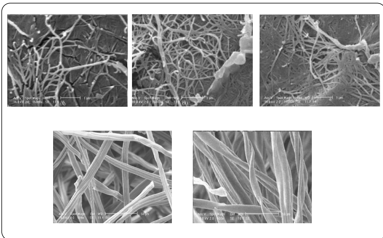
شکل ۹- تصویرهای میکروسکوپ الکترونی SEM سلولز باکتریایی تولید شده از الف) ساکاروز- با بزرگنمایی ۱۵۰۰۰X، ب) لاکتوز با بزرگنمایی ۱۵۰۰۰X، ج) گلوکز با بزرگنمایی ۱۵۰۰۰X، د) الیاف پنبه با بزرگنمایی ۵۰۰ X، ه) الیاف ویسکوز با بزرگنمایی ۵۰۰X
