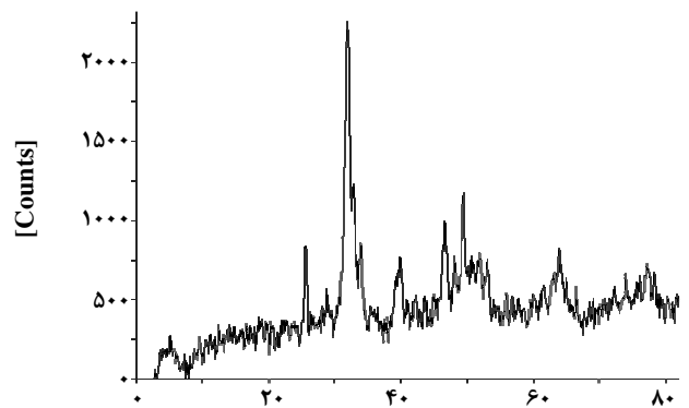
شکل ۵ - طیف XRD نمونه TCP-۱۰.
