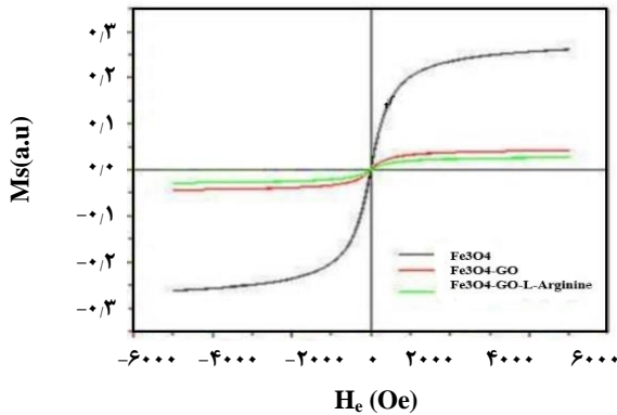
شکل ۷ - بررسی مغناطیس پذیری \text{Fe}_3\text{O}_4 ، \text{GO}/\text{Fe}_3\text{O}_4 و \text{GO}/\text{Fe}_3\text{O}_4/\text{L-Arginine} .
