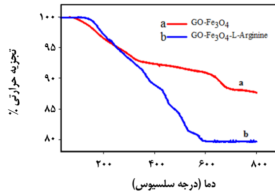
شکل ۶ - منحنی‌های تجزیه وزن سنجی حرارتی \text{GO}/\text{Fe}_3\text{O}_4 و \text{GO}/\text{Fe}_3\text{O}_4/\text{L-Arginine} .
