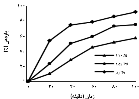
شکل ۹- بازده فرایند تخریب بر روی کاتالیست های انتخابی در شرایط اسیدی (غلظت رنگ: ۲۰ ppm، غلظت فوتوکاتالیست: ۲۰ ppm، دمای اتاق).
