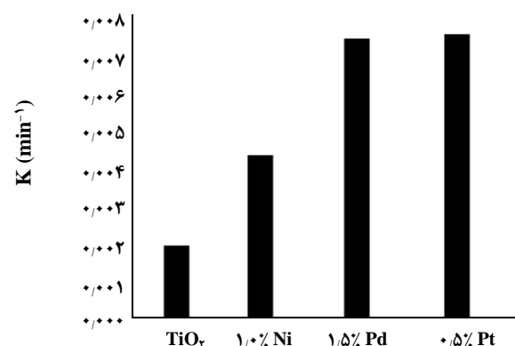
شکل ۱۱- تأثیر حضور فلزهای واسطه بر روی ثابت سرعت تخریب (غلظت رنگ: ۲۰ ppm، غلظت فوتوکاتالیست: ۲۰ ppm، pH=۷، دمای اتاق)
