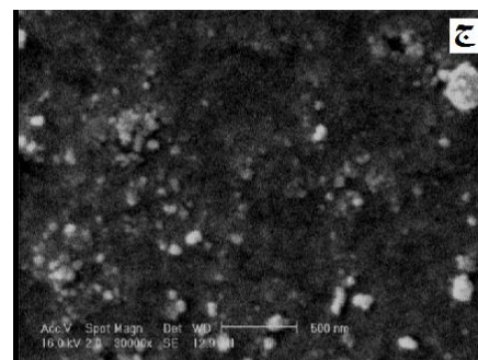
شکل ۴- تصاویر SEM فوتوکاتالیست‌های اصلاح شده با الف: Pt، ب: Pd و ج: Ni.
