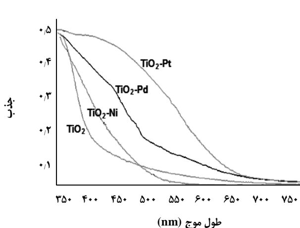
شکل ۶- طیف DRS فوتوکاتالیست‌های تهیه شده.
