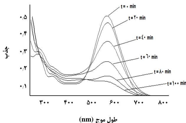
شکل ۷ - طیف جذبی رنگ AB92 بعد از ۱۰۰ دقیقه تخریب (غلظت رنگ: ۲۰ ppm، غلظت فوتوکاتالیست: ۲۰ ppm، pH=۷، دمای اتاق).
