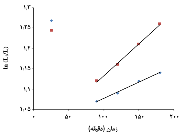
شکل ۶ - رابطه بین \ln(L_0/L) و زمان پخت در دمای ۲۰۰°C در شرایط استفاده از کاتالیست سدیم هیدروکسید ۲٪ و بدون آن.
