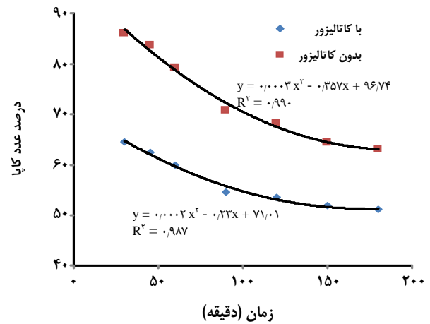
شکل ۱- رابطه بین عدد کاپا و زمان خمیر کاغذ سازی در دمای 200^{\circ}\text{C} و با استفاده از کاتالیزور هیدروکسید سدیم ۲٪ و بدون استفاده از آن.
