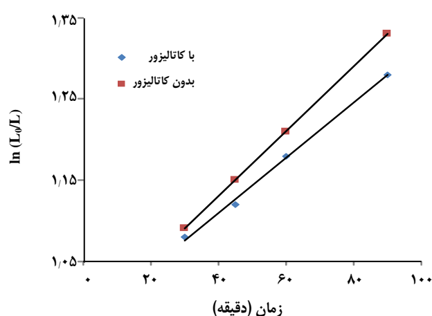
شکل ۵ - رابطه بین \ln(L_0/L) و زمان پخت در دمای ۲۰۰°C در شرایط استفاده از کاتالیزور سدیم هیدروکسید ۲٪ و بدون آن.
