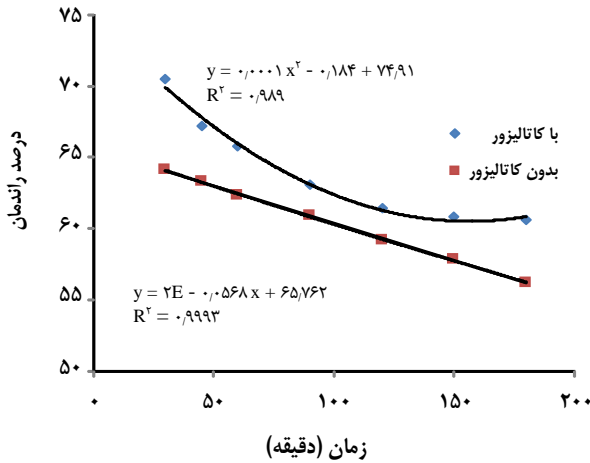
شکل ۲- رابطه بین راندمان و زمان خمیر کاغذ سازی در دمای 200^{\circ}\text{C} و با استفاده از کاتالیست سدیم هیدروکسید ۲٪ و بدون استفاده از آن.
