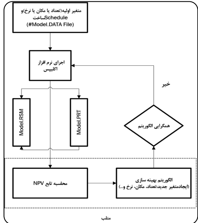
شکل ۳ - فلوچارت ارتباط بین متلب و شبیه‌ساز اکتیپس [۱۹]
