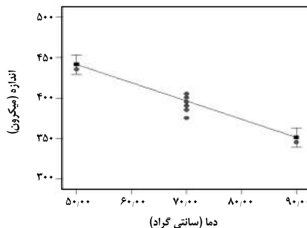
شکل ۱۰ - نمودار تغییرهای اندازه ذره-دما هوای ورودی.
