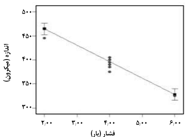
شکل ۱۱ - نمودار تغییرهای اندازه ذره-فشار هوای نازل.
