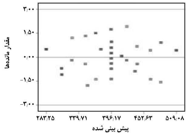
شکل ۷ - نمودار مقدار مانده‌ها در مقابل مقادیرهای پیش‌بینی شده اندازه ذره-میکرون.
