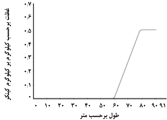
شکل ۶ - تغییر غلظت جز C_3S بر حسب طول ورودی کوره (از سمت پیش گرمکن).
