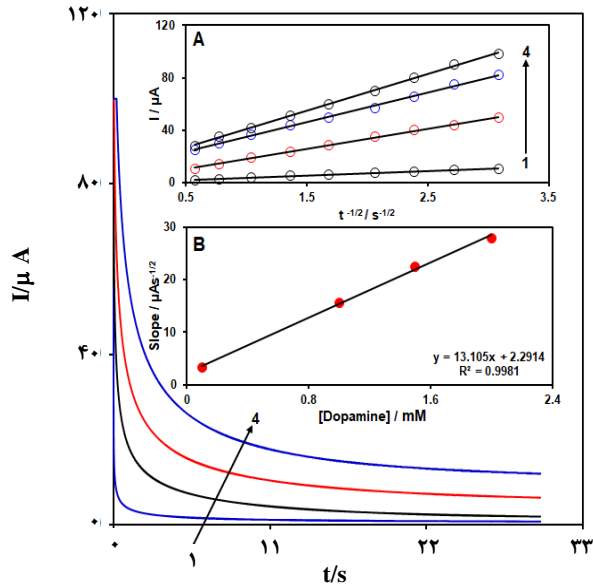
شکل ۶ - کروئوآمپروگرام‌های MnO_2/SPE در محلول بافر فسفات 0.1 M با pH=7.0 دارای غلظت‌های متفاوت (۱) 0.1 ، (۲) 1.0 ، (۳) 3.0 و (۴) 20.0 میلی مولار دوپامین. پله پتانسیل 300 mV می‌باشد. ضنائم: (A) تغییرهای I - t^{1/2} به دست آمده از کروئوآمپروگرام‌های ۱-۴ (B) نمودار شیب خطوط I - t^{1/2} بر حسب غلظت دوپامین.
