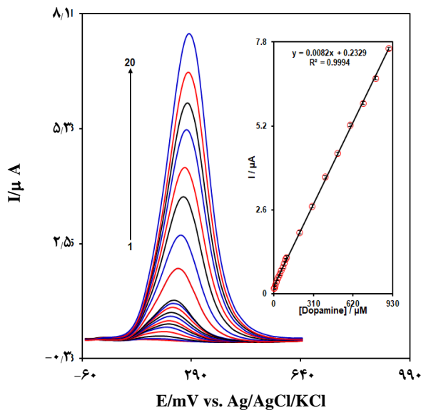
شکل ۷ - ولتاموگرام‌های پالس تفاضلی در محلول بافر فسفات 0.1 M با pH=7.0 در سطح MnO_2/SPE در غلظت‌های گوناگون دوپامین، شماره ۲۰-۱ به ترتیب مربوط به غلظت‌های 0.1 ، 1.0 ، 5.0 ، 10.0 ، 20.0 ، 30.0 ، 40.0 ، 50.0 ، 60.0 ، 70.0 ، 80.0 و 90.0 میکرومولار دوپامین در محلول بافر فسفات 0.1 M با pH=7.0 است. ضمیمه: منحنی تغییرهای جریان بر حسب غلظت دوپامین در بازه‌ی غلظتی 0.1-90.0 میکرومولار.
