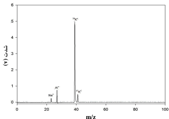
شکل ۳: طیف جرمی زمان پرواز صفحه آلومینیوم ثبت شده با تابش لیزر ۱۰۶۴ نانومتر و تاخیر زمانی Q-Switch ۳۵۰ میکرونانیه
