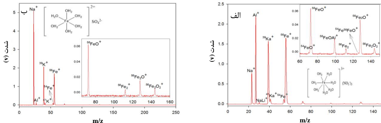
شکل ۵: طیف جرمی کمپلکس‌های الف) [\text{Fe}(\text{H}_2\text{O})_7](\text{NO}_3)_3 ، ب) [\text{Fe}(\text{H}_2\text{O})_6]\text{SO}_4 ثبت شده بر روی صفحه آلومینیوم
