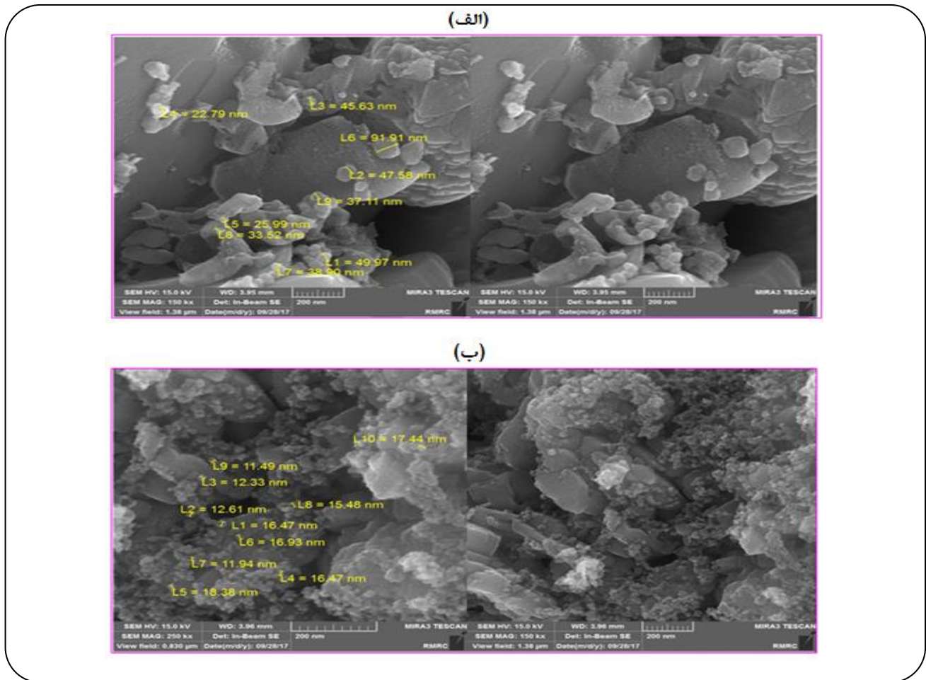
شکل ۶ - تصویرهای FESEM نانو ذره‌های (1) Cu NPs (الف) و (2) Cu NPs (ب).
