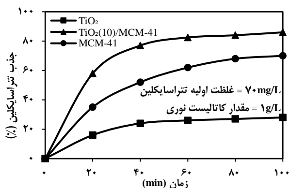
شکل ۹- نمودار میزان جذب سطحی تتراسایکلین بر حسب زمان
