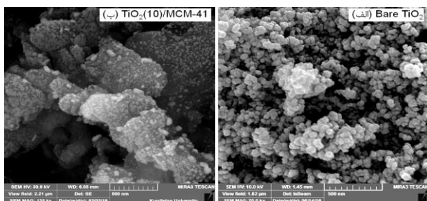
شکل ۵- تصویرهای آنالیز FESEM (الف) \text{TiO}_2 خالص و (ب) نانو چندسازه \text{TiO}_2/\text{MCM-41} سنتز شده
