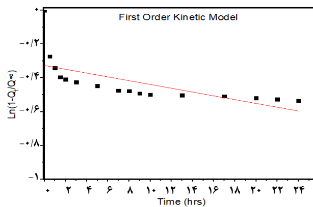
شکل ۱۰ - برازش داده‌های رهایش استامینوفن توسط حامل \text{Cu}_3(\text{BHTC})_2 در بافر فسفات سالین با مدل‌های سینتیکی متفاوت
