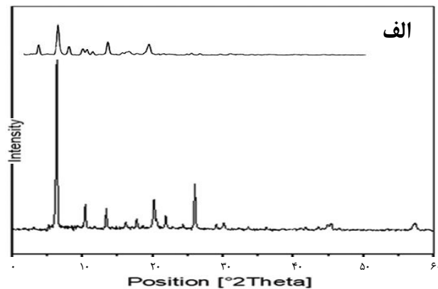
شکل ۷- الگوی پراش ایکس الف: \text{Fe}_1\text{Cu}_2(\text{BHTC})_2 ب: \text{Cu}_3(\text{BHTC})_2
