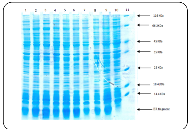
شکل ۱- تجزیه SDS-PAGE مربوط به نتیجه‌های طراحی تاگوچی. ستون‌های ۱-۹: نتیجه آزمایش‌های شماره ۱-۹ (مطابق جدول ۶)، ستون ۱۰ نمونه کنترل (القا نشده) و ستون ۱۱: شاخص وزن مولکولی.
