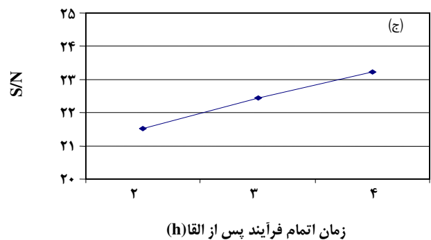
شکل ۲- منحنی S/N برای متغیرهای اصلی در طراحی تاگوچی: (الف) دما، (ب) زمان القا و (ج) زمان پایان فرایند.
