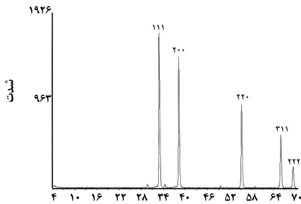
شکل ۴- الگوی پراش اشعه X برای نمونه کادمیم اکسید آلیش شده با ۱ درصدوزنی گادولینیوم.
