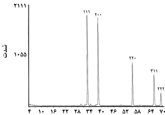
شکل ۵- الگوی پراش اشعه X برای نمونه کادمیم اکسید آلیش شده با ۴ درصدوزنی لوتیتیوم.
