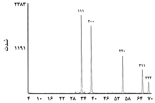
شکل ۱- الگوی پراش اشعه X برای کادمیم اکسید خالص.
