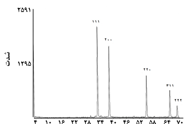
شکل ۲- الگوی پراش اشعه X برای نمونه کادمیم اکسید آلیش شده با ۴ درصدوزنی گادولینیوم.
