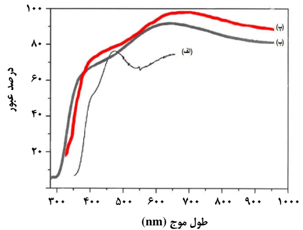
شکل ۱۳- طیف UV-Vis نمونه CdO تهیه شده به روش سل - ژل (الف) نمونه کادمیم اکسیدخالص (ب) آلاینش شده با ۰٫۸ درصد وزنی Gd (پ) آلاینش شده با ۰٫۸ درصد وزنی Lu.
