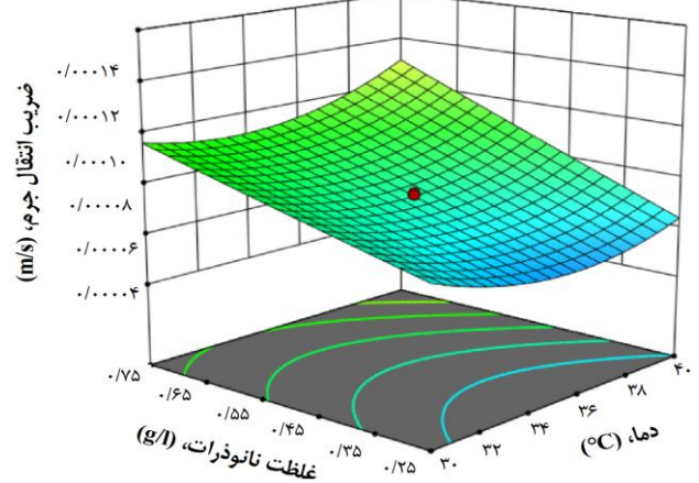
شکل ۸- اثر دما و غلظت نانو ذره‌ها بر ضریب انتقال جرم فاز مایع در شدت جریان 200 \text{ ml/min}
