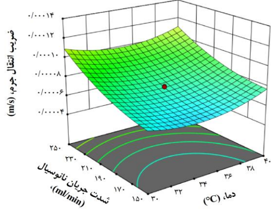
شکل ۹- اثر جریان و دما بر میزان ضریب انتقال جرم. با k_L غلظت ثابت ۰/۵ g/l
