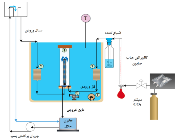
شکل ۱- طرح‌واره کلی از برج دیواره مرطوب: ۱: WWC، ۲: کویل، ۳: هیتر، ۴: پمپ.
