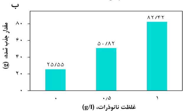
شکل ۵- نرخ جذب کربن دی‌اکسید در آب و نانوسیال در دمای ۳۵ °C و شدت جریان ۲۰۰ ml/min
