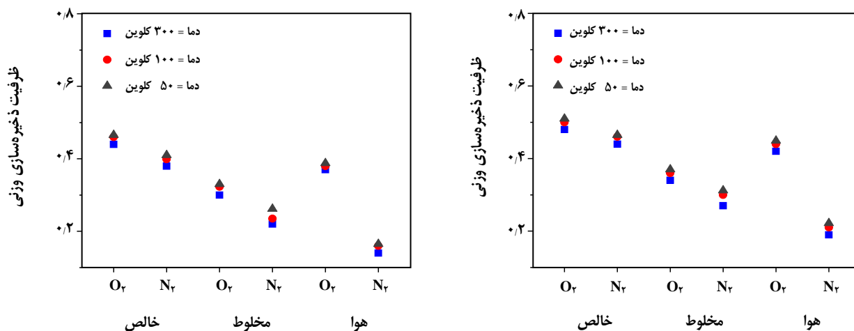
نمودار ۵ - ظرفیت ذخیره‌سازی وزنی (الف) نانومخروط و (ب) نانولوله کربنی در دماهای گوناگون.
