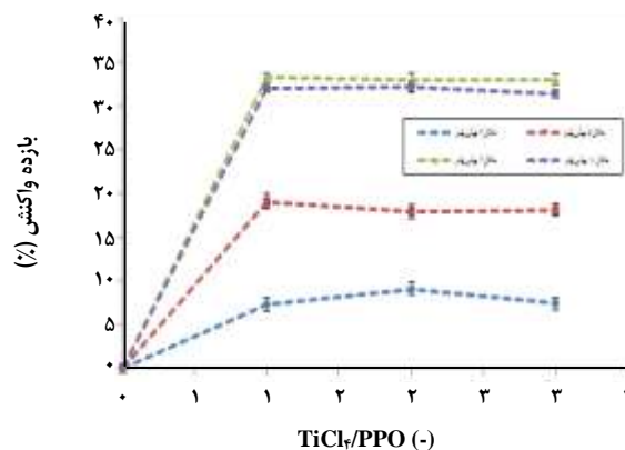
شکل ۲- بازده واکنش کوپلیمریزاسیون پلی اتر با فنیل ایزوسیانات بر حسب نسبت \text{TiCl}_4/\text{PPO} در مقادیر گوناگون حلال (زمان واکنش ۱ ساعت، دمای واکنش ۲۵ °C و میزان فنیل ایزوسیانات ۲۰ mmol).
