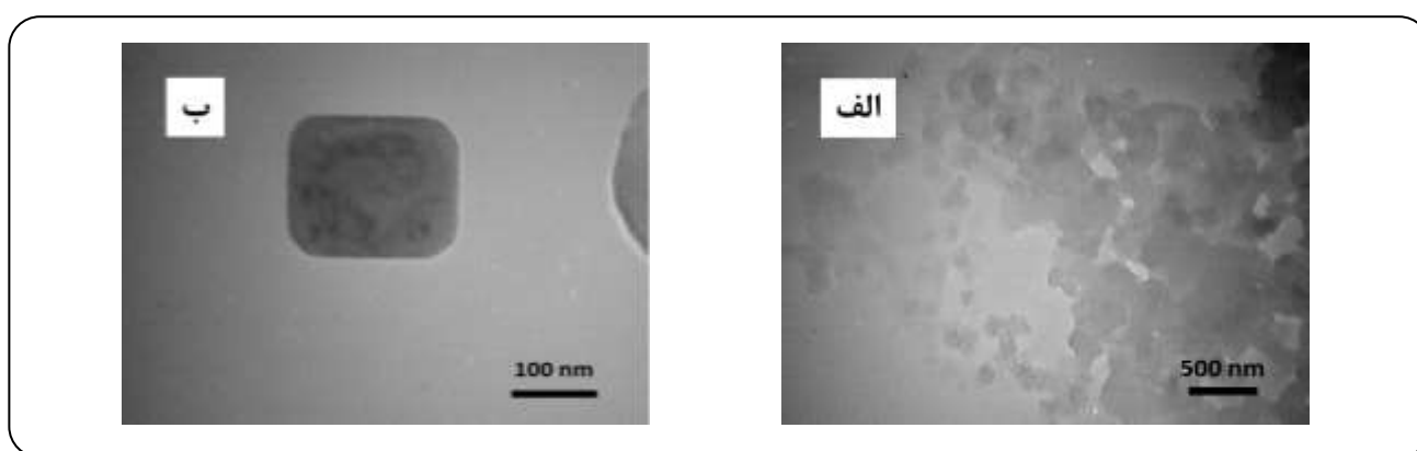
شکل ۸ - تصویر TEM (الف) مجموعه‌ای از ذره‌های مکعبی کوپلیمر پلی اتر - قطعه - پلی فنیلن ایزوسیانات پس از ۲ ساعت آسیاب با مقیاس ۵۰۰ nm، (ب) تصویر ذره کوپلیمر سنتز شده با مقیاس ۱۰۰ nm.
