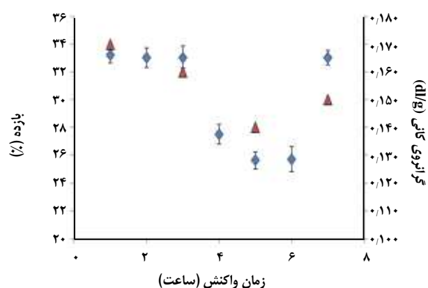
شکل ۳- نمودار بازده واکنش (علامت لوزی) و گرانیوی (علامت مثلث) کوپلیمریزاسیون بر حسب زمان در حضور کاتالیست TiCl_4 (دمای واکنش 25^{\circ}C ، نسبت TiCl_4/PPO برابر با ۱، ۷ ml تولوئن و میزان فنیل ایزوسیانات ۲۰ mmol).
