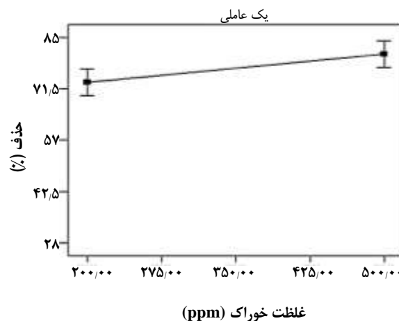
شکل ۷ - اثر غلظت خوراک بر میزان حذف سختی در شرایط بهینه به دست آمده از نرم افزار.
