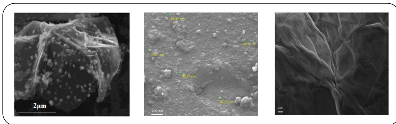
شکل ۴- تصویر FE-SEM گرافن اکسید (آ)، نانوذره‌های آهن اکسید (ب) و نانوکامپوزیت آهن اکسید/ گرافن (ج).
