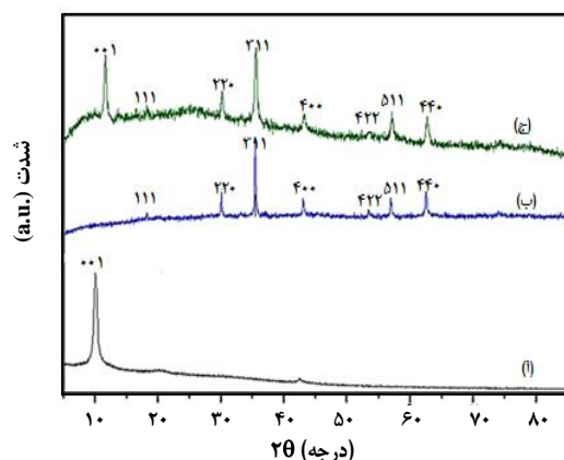
شکل ۳- الگوی XRD گرافن اکسید (آ)، نانوذرات آهن اکسید (ب) و نانوکامپوزیت آهن اکسید/ گرافن (ج).
