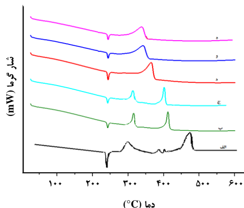
شکل ۵ - منحنی تجزیه گرمایی تجزیه DSC (الف) آمونیوم پرکلرات خالص (ب) آمونیوم پرکلرات + ۵٪ گرافن اکسید (ج) آمونیوم پرکلرات + ۵٪ آهن اکسید (د) آمونیوم پرکلرات + ۲٪ نانوکامپوزیت آهن اکسید/ گرافن (و) آمونیوم پرکلرات + ۴٪ نانوکامپوزیت آهن اکسید/ گرافن (ه) آمونیوم پرکلرات + ۵٪ نانوکامپوزیت آهن اکسید/ گرافن.
