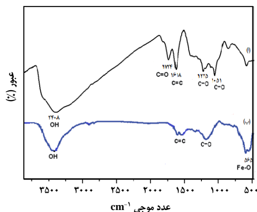
شکل ۲- طیف FT-IR گرافن اکسید (آ) و نانوکامپوزیت آهن اکسید/ گرافن (ب).
