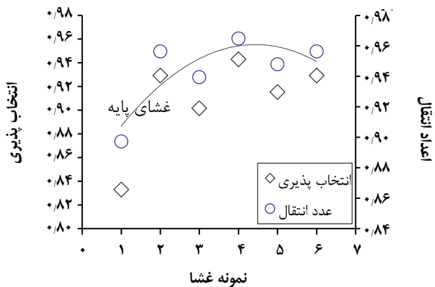
شکل ۶- انتخاب پذیری و عدد انتقال غشاهای تبادل کاتیونی تهیه شده با نسبت های گوناگونی از اختلاط پلیمرهای پایه پلی وینیل کلراید/پلی اتیلن گلايکول.
