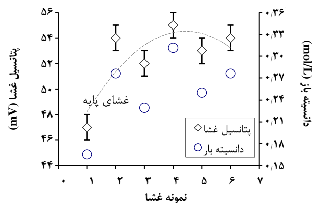
شکل ۵- اثر پلی اتیلن گلايکول در ساختار غشاها بر پتانسیل و دانسیته بار.
