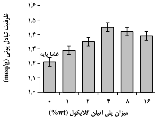
شکل ۴- ظرفیت تبادل یونی غشاهای تبادل کاتیونی: بررسی اثر میزان پلی اتیلن گلیکول در ساختار غشا.
