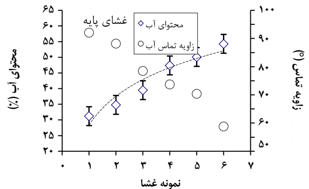
شکل ۳- اثر افزایش میزان پلی اتیلن گلیکول بر محتوای آب و زاویه تماس سطحی غشاهای تهیه شده.
