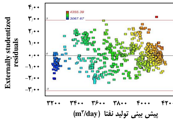
شکل ۱۰- نمودار باقیمانده بر حسب مقدار پیش بینی شده برای نفتای سبک و سنگین.
