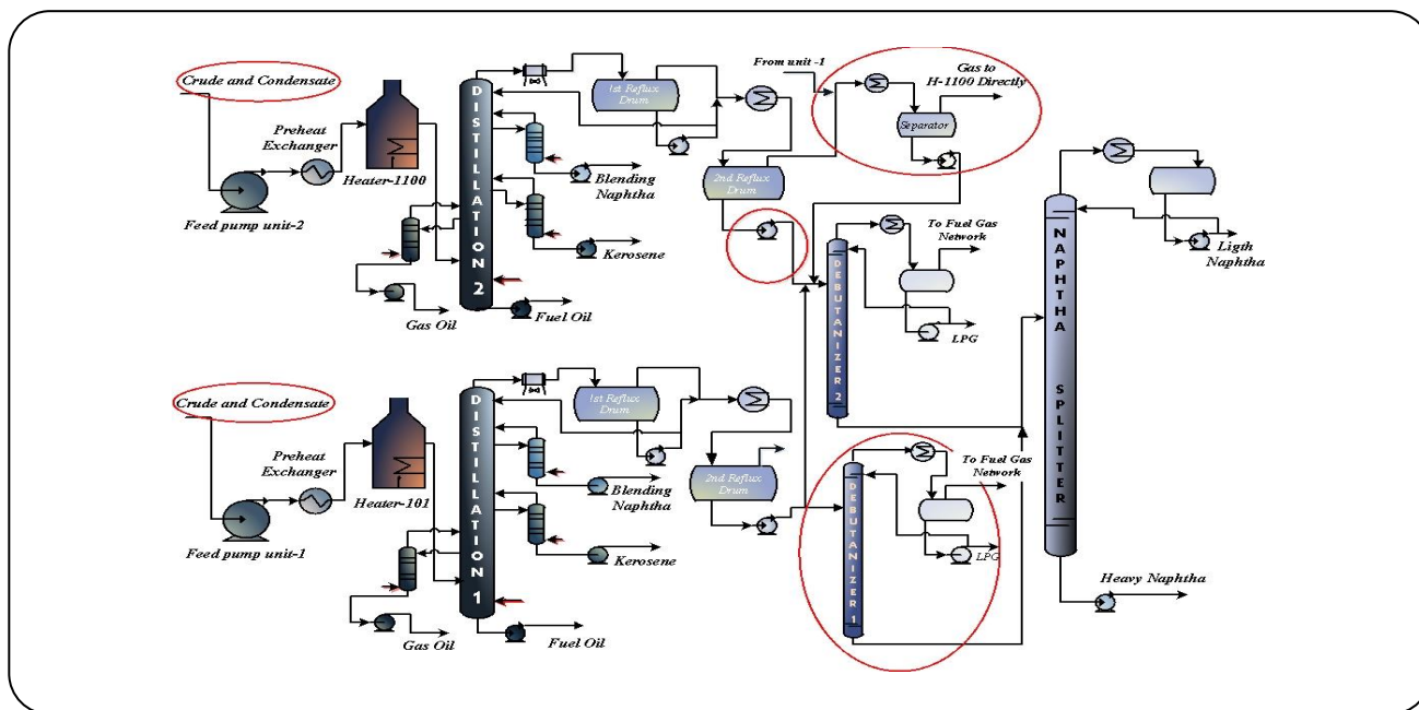
شکل ۱۷- شمای از واحد تقطیر پالایشگاه لاوان پس از اعمال تغییرهای فرایندی برای دستیابی به شرایط بهینه.
