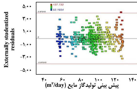
شکل ۹- نمودار باقیمانده بر حسب مقدار پیش بینی شده برای گاز مایع.
