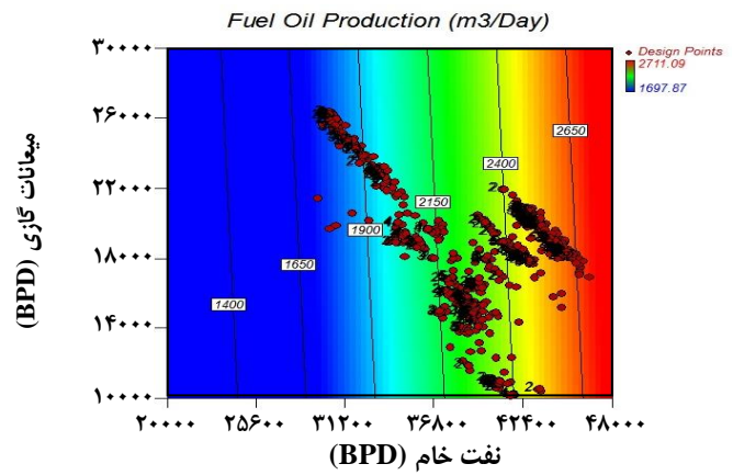
شکل ۱۶ (الف و ب) - تأثیر همزمان مقدار نفت خام و میعان های گازی بر روی مقدار نفت کوره تولیدی.
