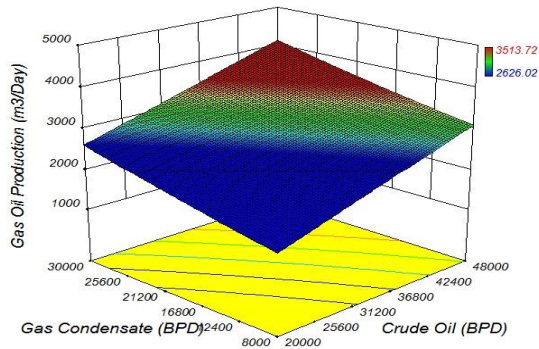
شکل ۱۵ (الف و ب) - تأثیر همزمان مقدار نفت خام و میعان های گازی بر روی مقدار نفت گاز تولید.
