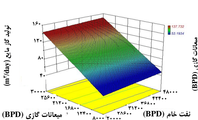
شکل ۱۳ (الف و ب) - تأثیر همزمان مقدار نفت خام و میعان‌های گازی بر روی مقدار گازمیع تولیدی.
