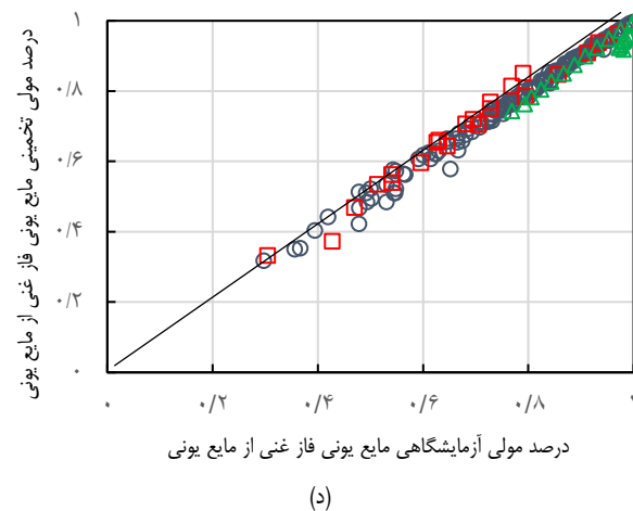
شکل ۵- نمایش کسر مولی تخمین‌زده با واقعی با استفاده شبکه MLP، (الف) ترکیب آلیفاتیک در فاز غنی از آلکان (ب) ترکیب آروماتیک در فاز غنی از آلکان (ج) ترکیب آروماتیک در فاز غنی از مایع یونی (د) ترکیب مایع یونی در فاز غنی از مایع یونی که در آن نقطه‌های با علامت (○) داده‌های آموزشی، نقاط با علامت (□) داده‌های اعتبارسنجی و نقاط با علامت (△) داده آزمایشی است.
