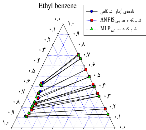
(الف) [Omim][SCN] ۰.۰ ۰.۱ ۰.۲ ۰.۳ ۰.۴ ۰.۵ ۰.۶ ۰.۷ ۰.۸ ۰.۹ ۱.۰ Hexane
