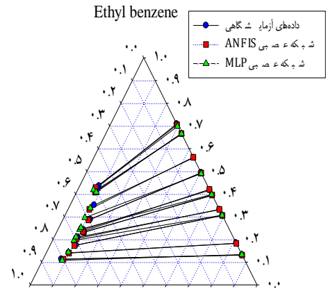
(ب) [Omim][SCN] ۰.۰ ۰.۱ ۰.۲ ۰.۳ ۰.۴ ۰.۵ ۰.۶ ۰.۷ ۰.۸ ۰.۹ ۱.۰ Heptane
