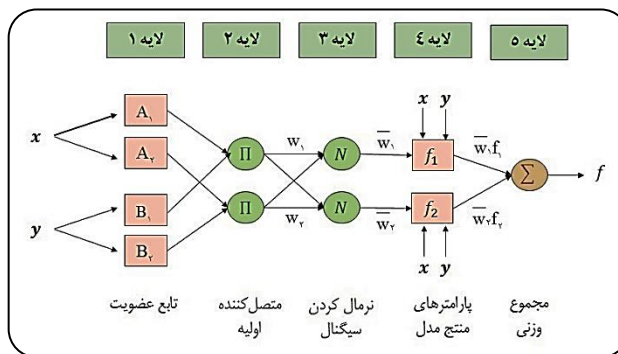
شکل ۱- ساختار مدل ANFIS با دو ورودی، یک خروجی و دو جدول قوانین [۴۱].
