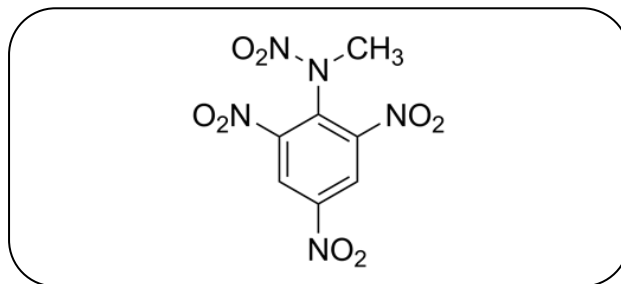
شکل ۱- ساختار شیمیایی تتریل.
