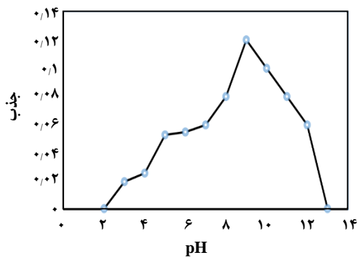
شکل ۳ - بررسی اثر pH محلول بر روی جذب تتریل. شرایط استخراج: حجم محلول آبی، ۱۰ mL؛ غلظت تتریل، ۱۰۰ ng/mL؛ حجم CCl_4 دارای آلکوات، ۲۰۰ \mu L؛ زمان هم‌زدن، ۵ ثانیه؛ زمان سانتریفیوژ، ۵ دقیقه
