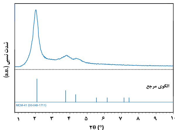
شکل ۳ - آنالیز XRD پایه سیلیکایی MCM-41 سنتز شده
