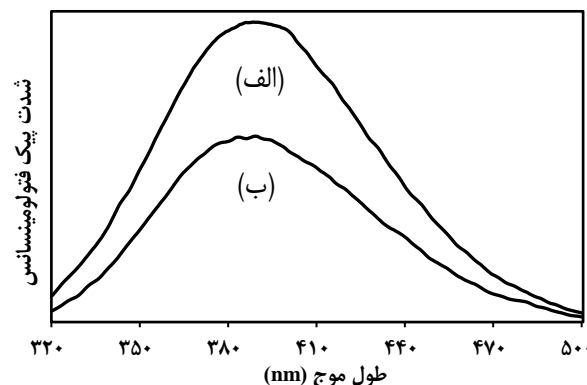
شکل ۷ - نمودار شدت پیک PL بر حسب طول موج (الف) \text{TiO}_2 خالص و (ب) نانو چندسازه \text{TiO}_2/\text{MCM-41} سنتزی
