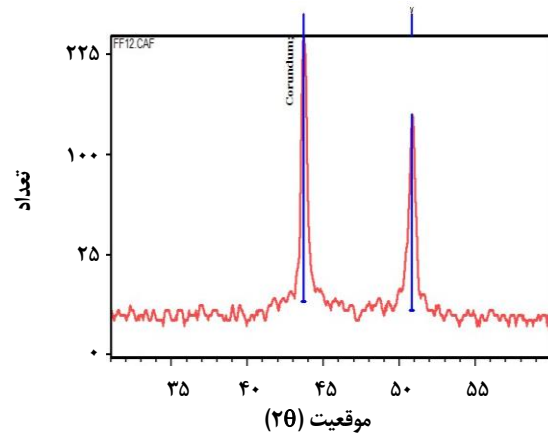
شکل ۴ - طیف XRD برای نمونه با زیر لایه فولاد ضد زنگ.
