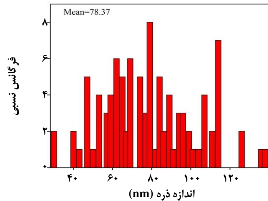
شکل ۱۰- هیستوگرام توزیع ابعاد دانه های نشانده شده با گاز نیتروژن.
