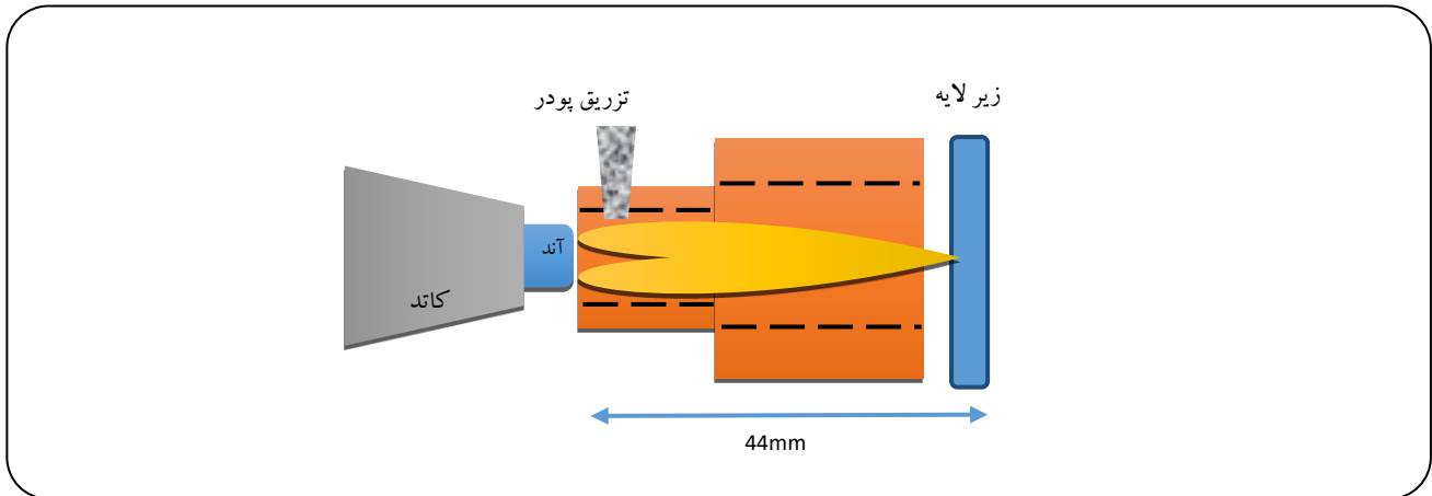
شکل ۱- طرحواره مشعل پلاسمایی.
