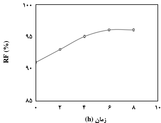
شکل ۵- فاکتور جداسازی در زمان‌های طولانی در دمای ۴۰ درجه سلسیوس و اختلاف فشار ۲ بار.
