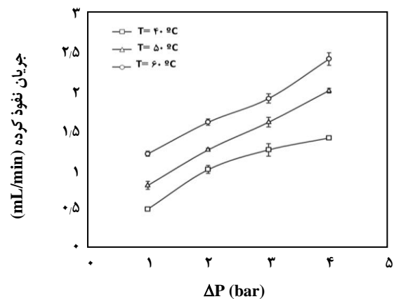
شکل ۴- شدت جریان عبور کرده از غشا در دماها و اختلاف فشارهای گوناگون دو سمت غشا.
