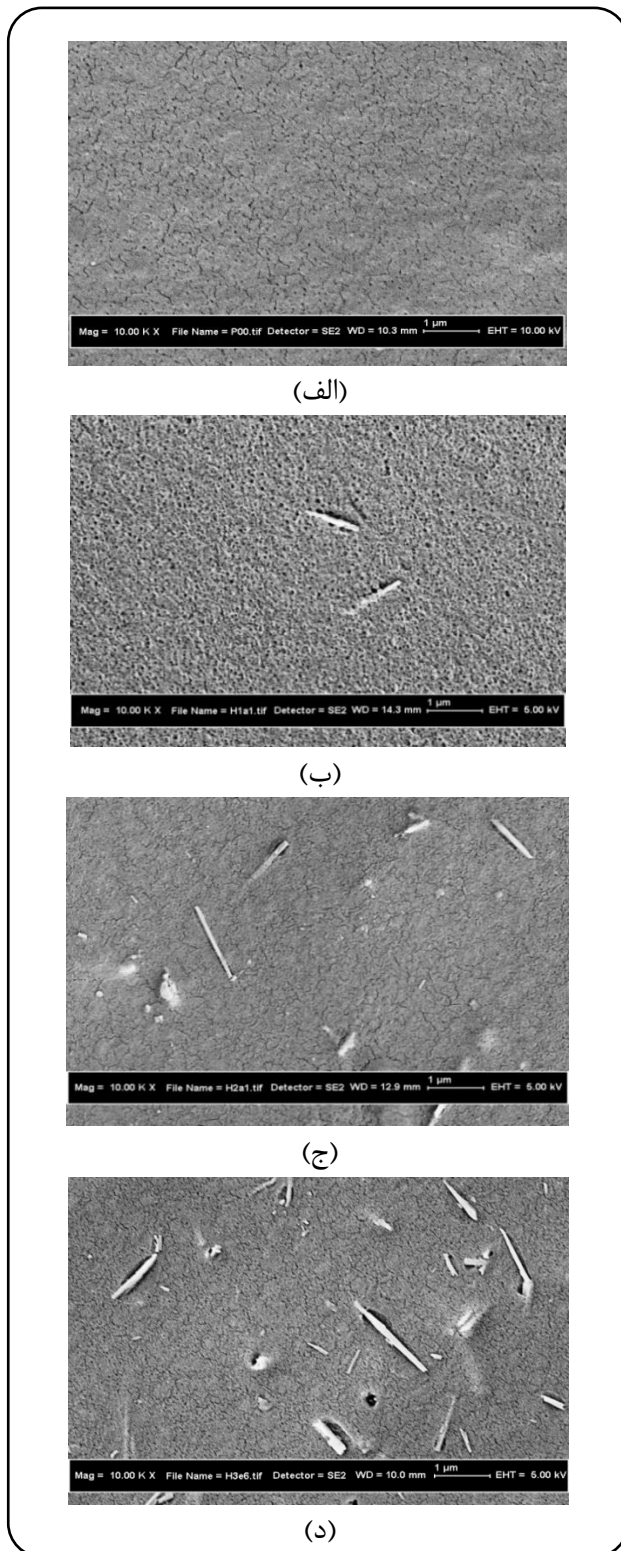
شکل ۴ - تصویرهای SEM از ساختار سطحی غشای (الف) غشای کنترل (ب) نانوکامپوزیت mHNT ۰.۲۵ (ج) نانوکامپوزیت mHNT ۰.۵ (د) نانوکامپوزیت mHNT ۱
