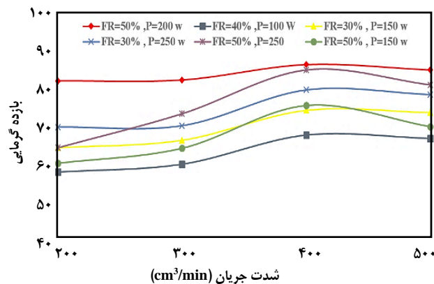
شکل ۵. تغییر بازده بر حسب شدت جریان در A.R=20
