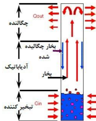
شکل ۱. طرح‌واره عملکرد ترموسیفون
