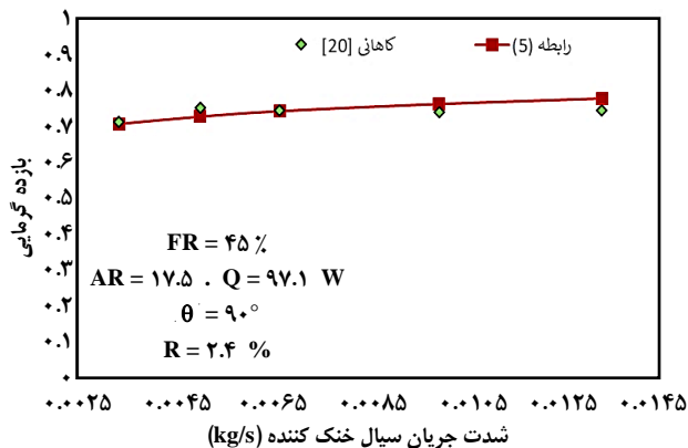
شکل ۸. مقایسه مرجع [۲۰] و رابطه (۵) در نسبت پر شدن ثابت
