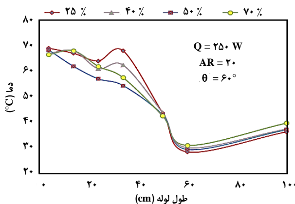
شکل ۷. توزیع دما در ترموسیفون در Q=250\text{ W} , \theta=60^\circ , A.R=20
