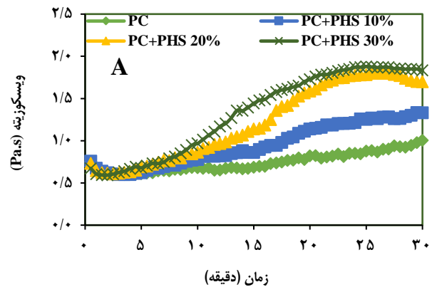
شکل ۵ - تأثیر مقدار سرباره بر گرانیوی در شدت برش ثابت 5 \times 10^{-1} (A): سیمان آمیخته دارای ۱۰، ۲۰ و ۳۰٪ سرباره فسفر، (B): سیمان آمیخته دارای ۱۰، ۲۰ و ۳۰٪ سرباره ذوب آهن
