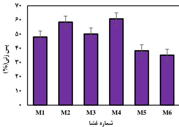
شکل ۸ - تغییرات پس‌زنی نمک سدیم سولفات در غلظت‌های گوناگون نانوذره‌ها برای غشاهای تهیه شده
