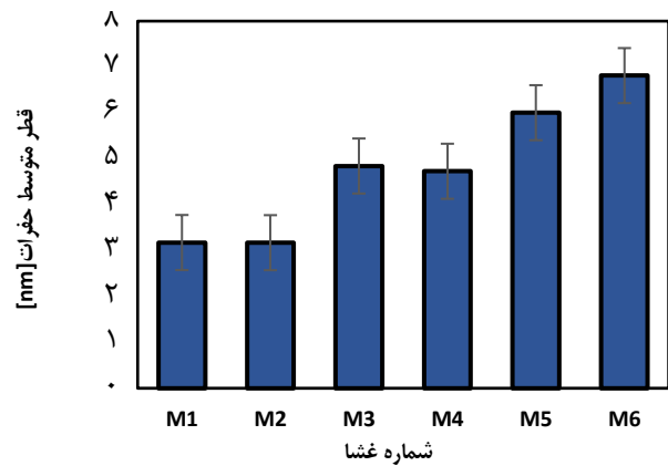
شکل ۶ - تغییرات قطر متوسط روزنه‌ها با تغییر غلظت نانوذره‌ها در ساختار غشا
