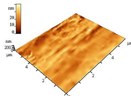
M_1 , R_a=10.12 \text{ nm}
